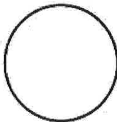
Cirkel Alla punkter på cirkeln lika långt ifrån centrum av cirkeln.
