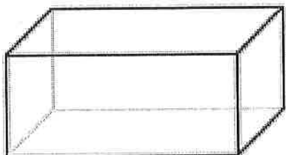
Rätblock Består av sex parvis likadana rektanglar.
