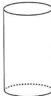
Cylinder Består av två parallella bottenytor i form av cirklar som är sammanbundna med en mantelyta.
