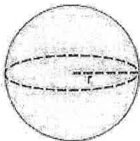
Klot Alla punkter på klotets yta ligger lika långt ifrån klotets centrum.
