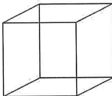
Kub Består av sex likadana kvadrater.
