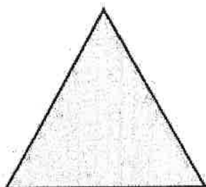
Triangel Tre hörn
