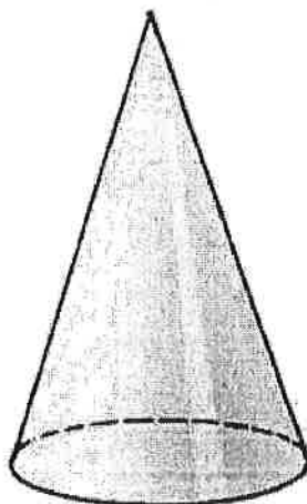
Kon Bottenytan är en cirkel. Mantelytan avslutas i en spets.
