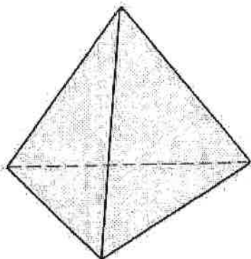
Tetraeder Består av fyra likadana trianglar.
